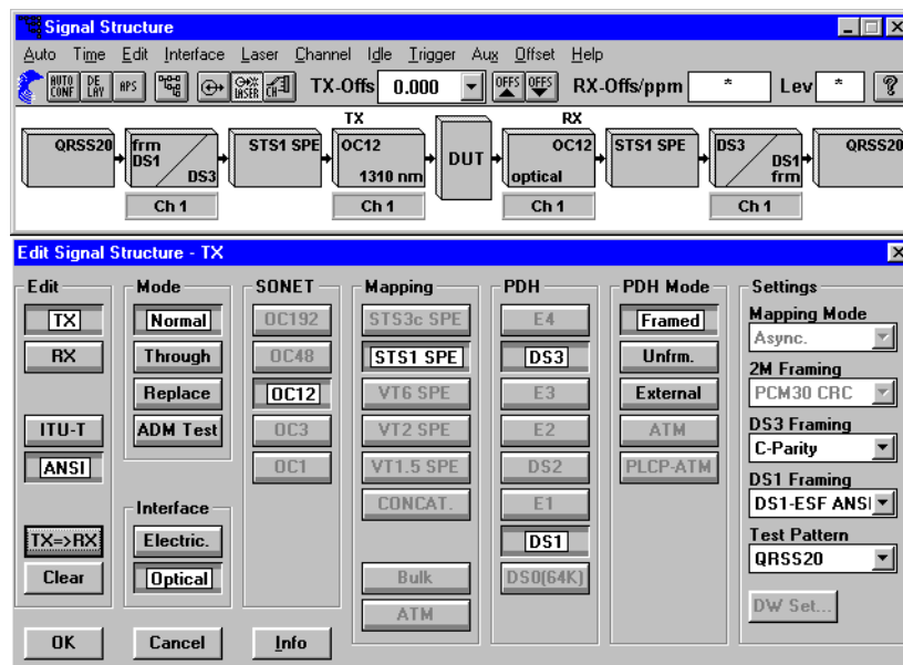
Bild E-1 Test eines Add-Drop-Multiplexers (ADM) mit M13-Multiplexer
